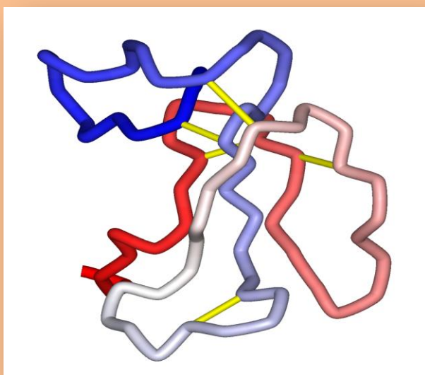
Molekula strupa črne mambe, ki lahko povzroči smrt.
